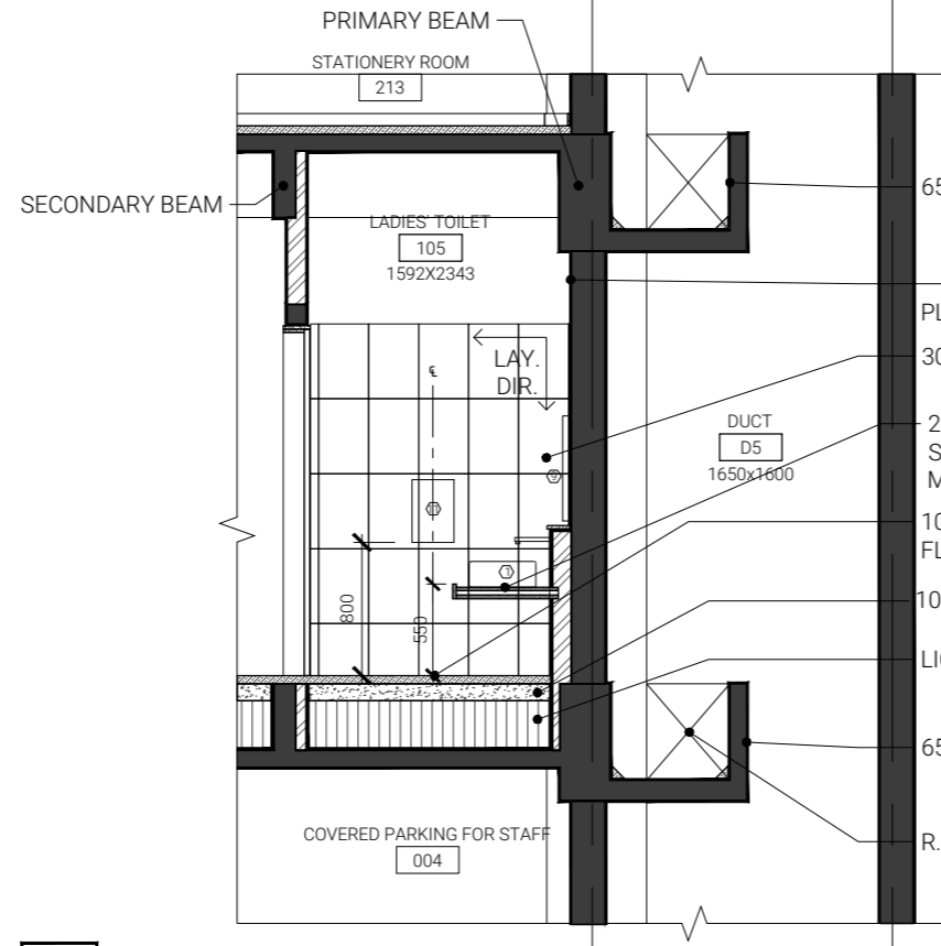
4 ELEVATION 11 1:50
