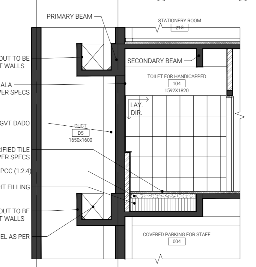
6 ELEVATION 13 1:50
