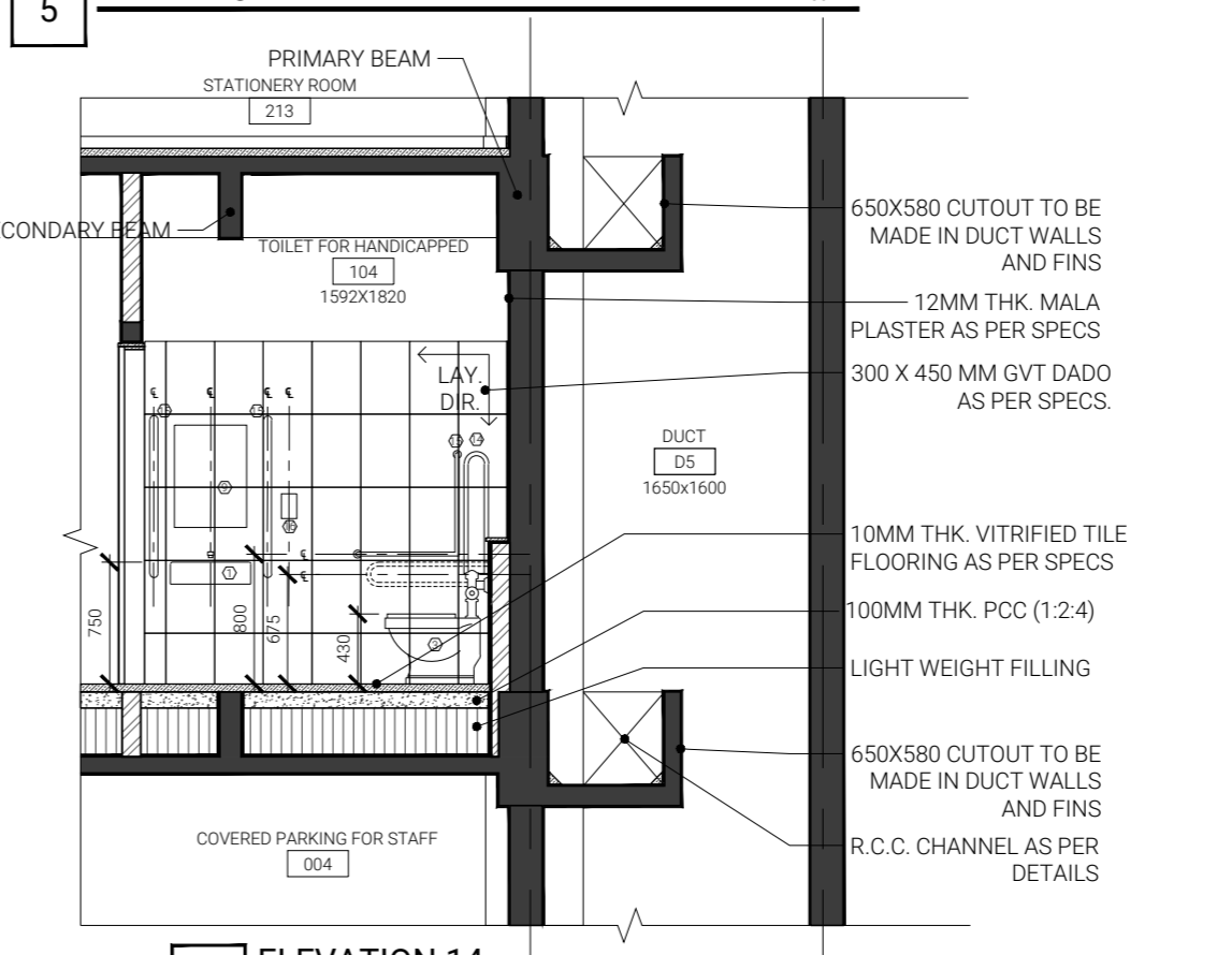
3 ELEVATION 14 1:50
