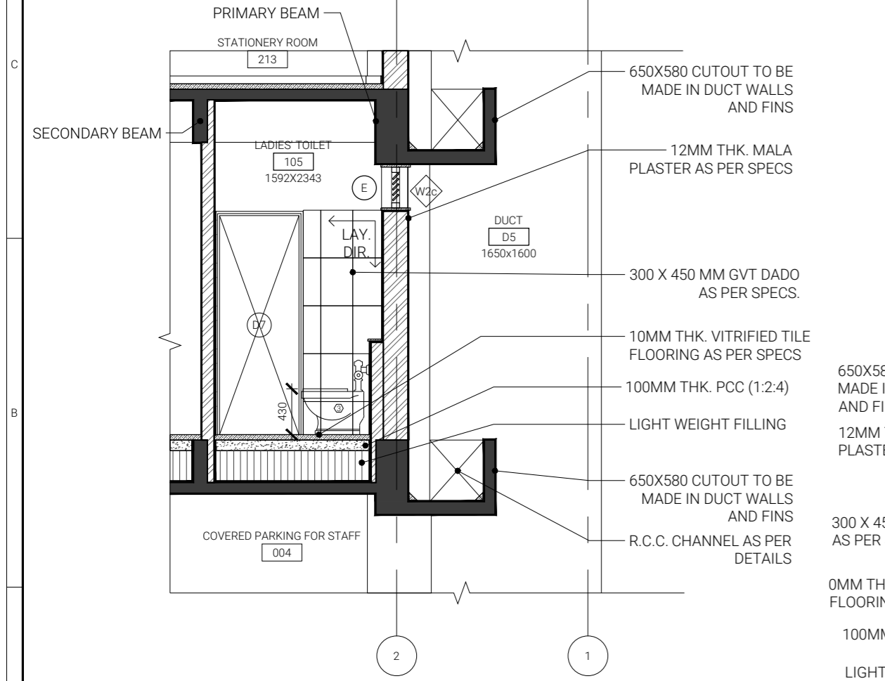
3 ELEVATION 10 1:50
